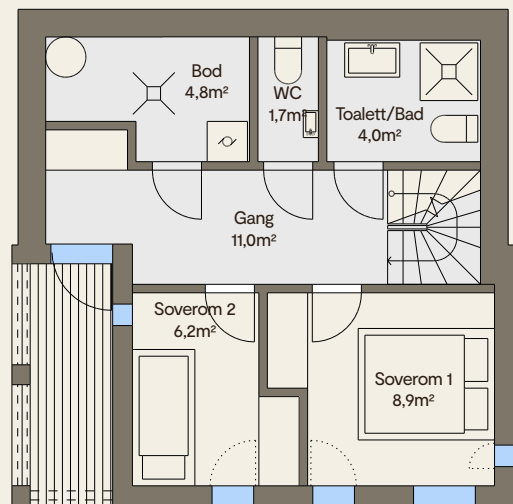
Plan underetasje
