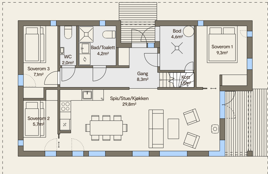
Plan hovedetasje
