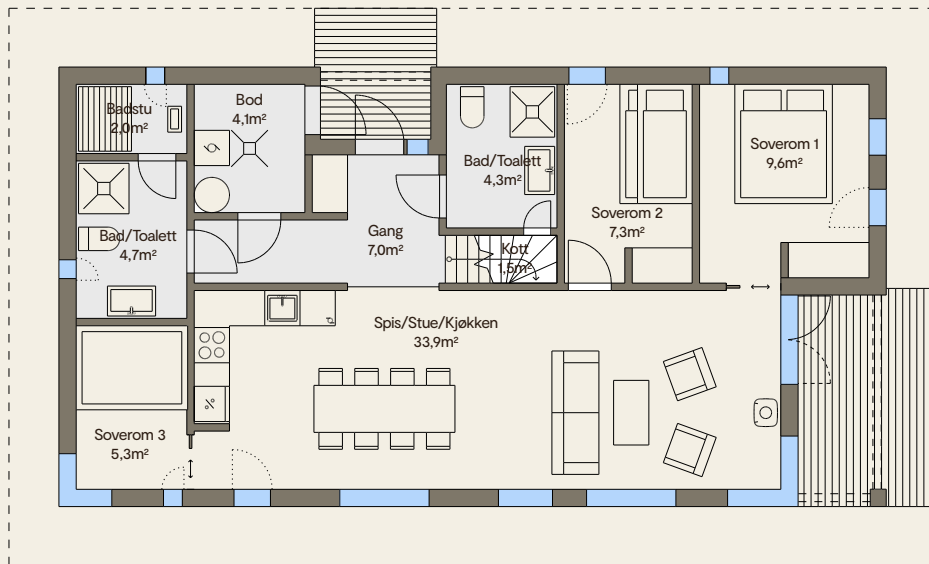
Plan hovedetasje
