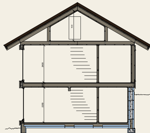
Snitt
