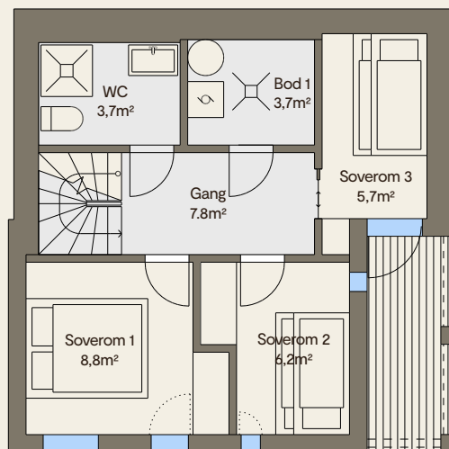
Plan underetasje
